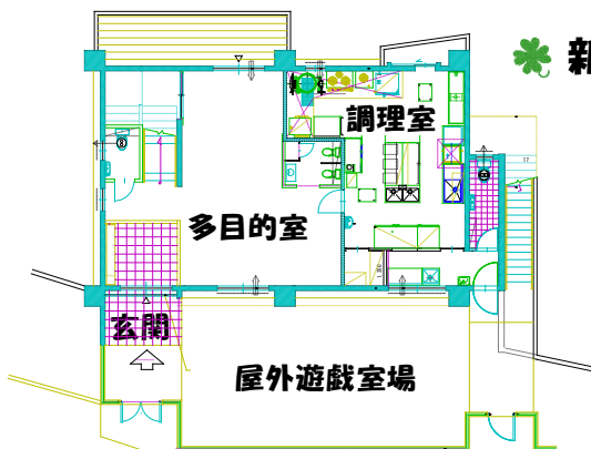
1階平面図
